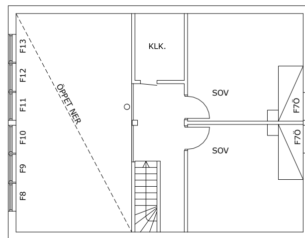
LOFTPLAN
